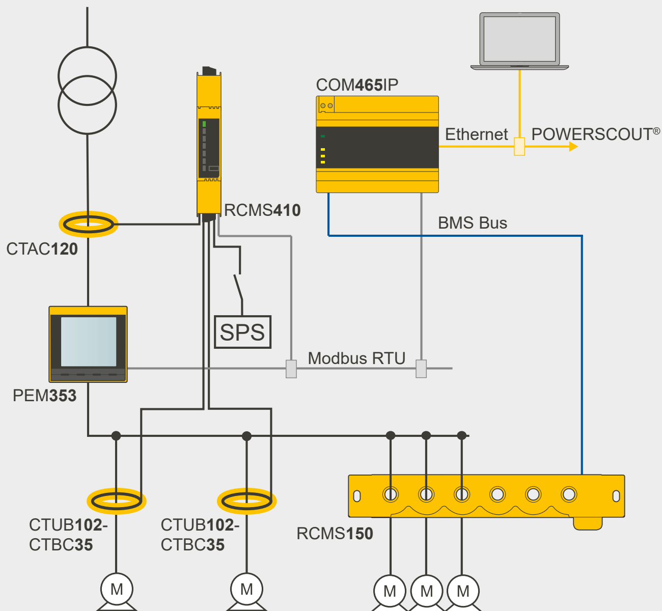
Systembeispiel für die Überwachung einer elektrischen Anlage
